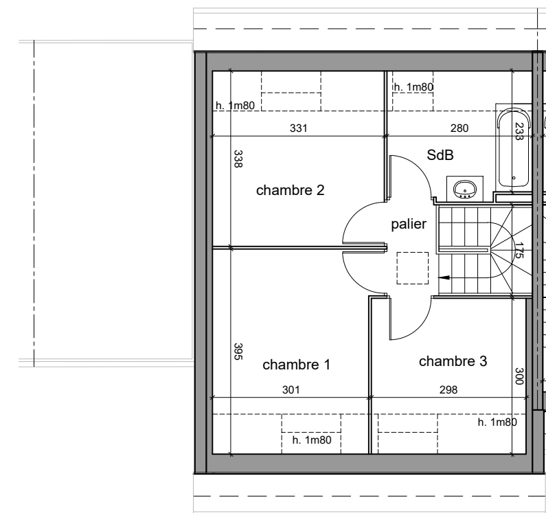
PLAN DE L'ETAGE
