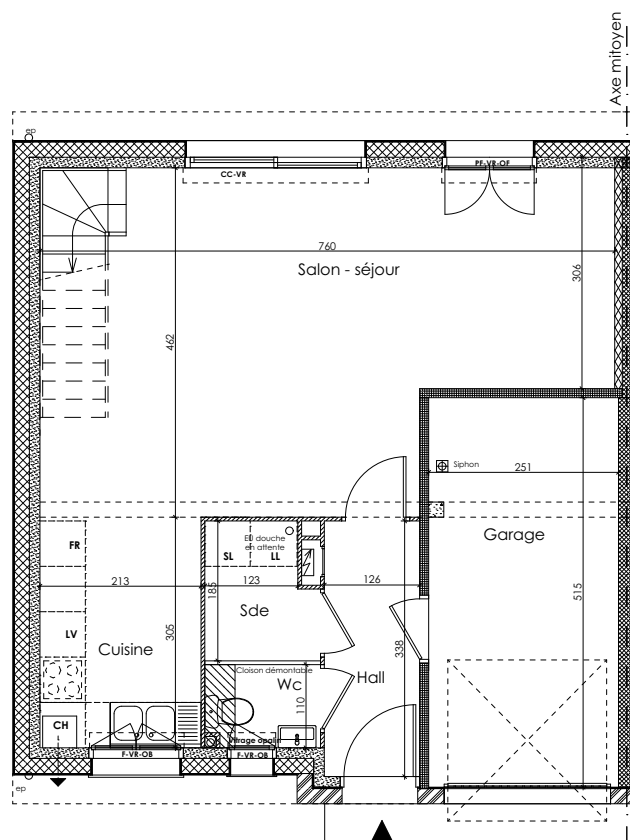
RDC 1:100
