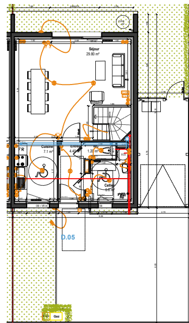
Plan du rez-de-chaussée
