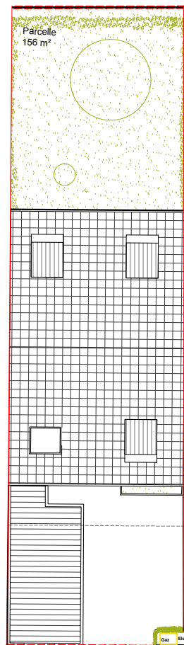
Plan du rez-de-chaussée
