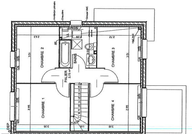
ETAGE
