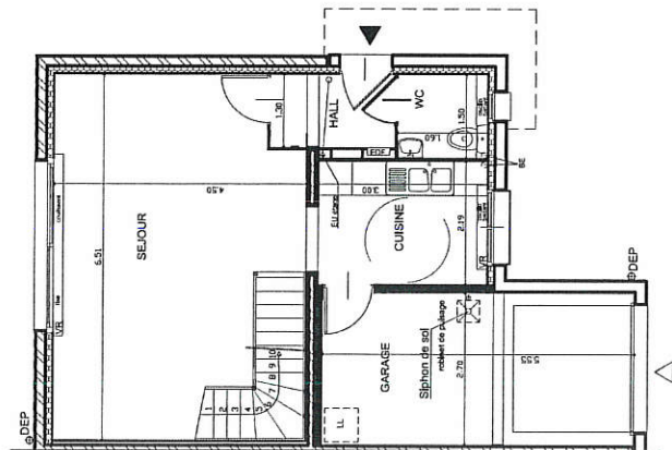
REZ-DE-CHAUSSEE
